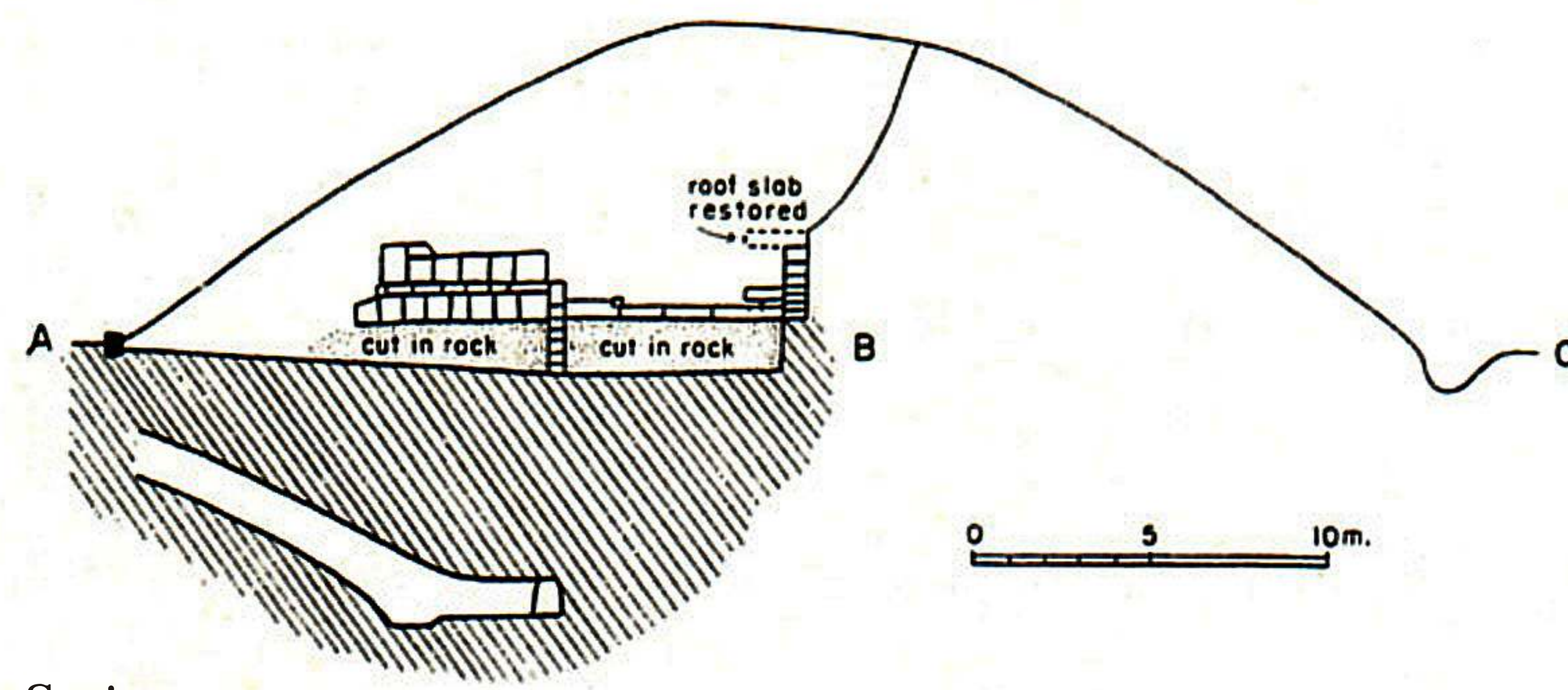
Sezione
