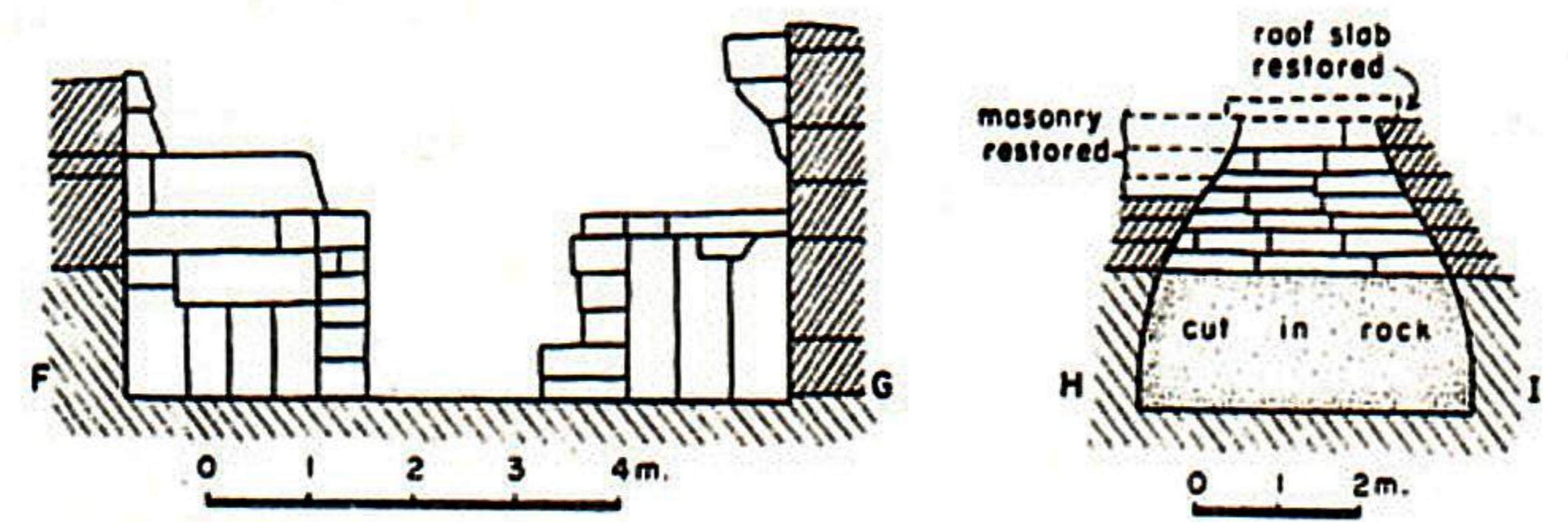
Prospetti
